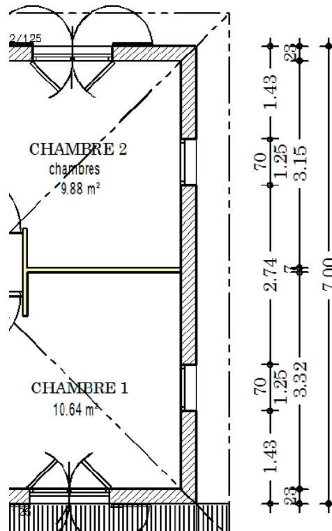
Figure 5-Détail de la paroi extérieure Nord de l'étage
