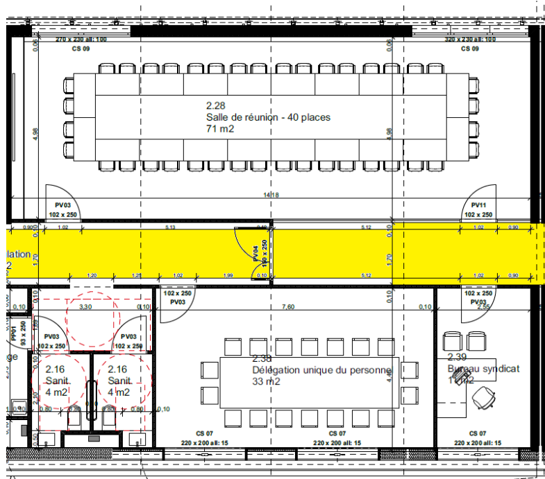
Circulations (en jaune) intégrées à la zone bureaux
