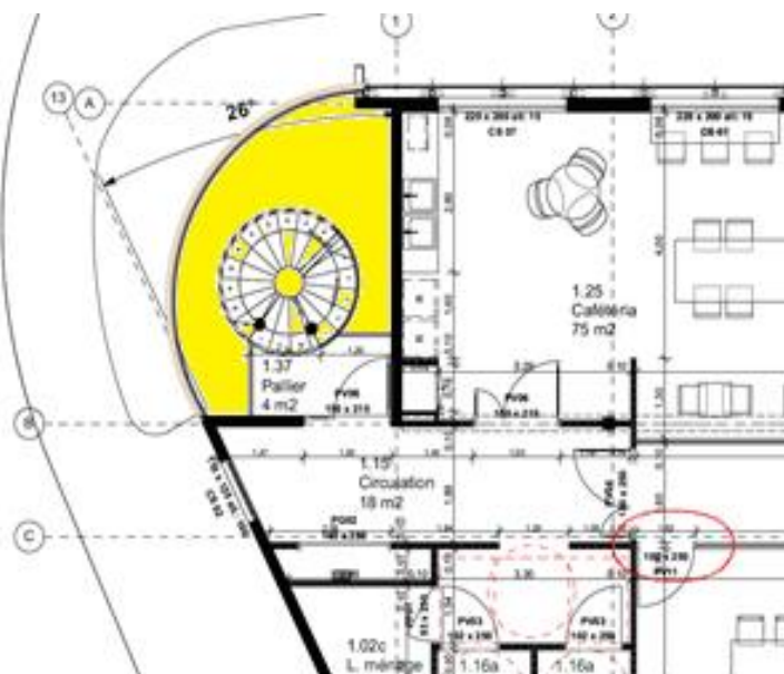
Vue extérieure et sur plan (partie jaune) des coursives des différents étages.
