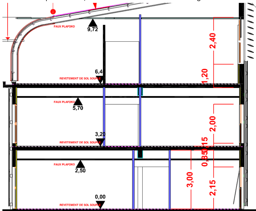
Vue en coupe du bâtiment
