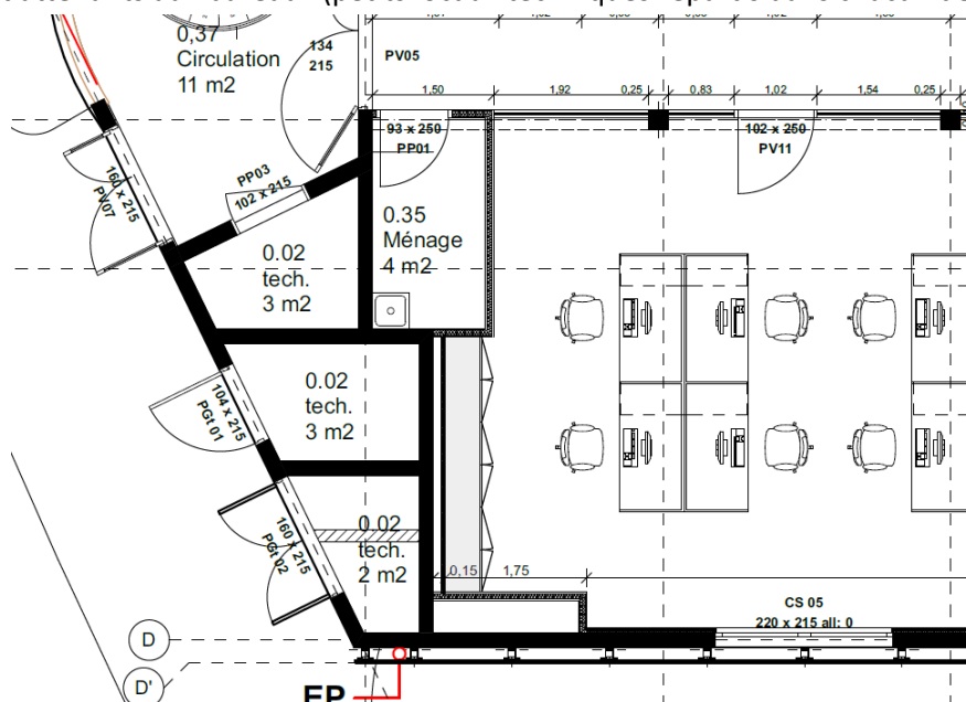
Détail montrant le positionnement des locaux techniques dans le bâtiment
