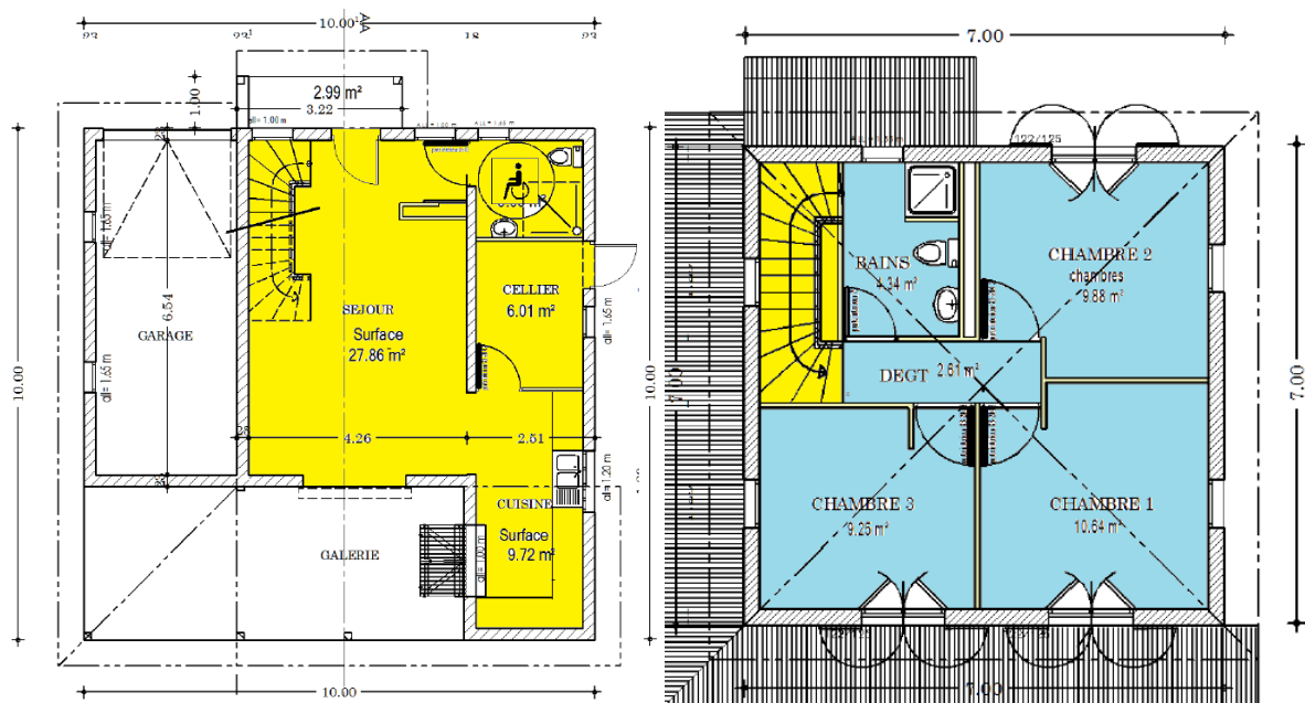
Figure 4- Répartition des différentes pièces de la maison entre zone jour (jaune) et nuit (bleu)
